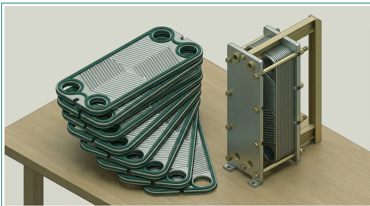
Подбор аналога Sondex по типоразмеру пластины
