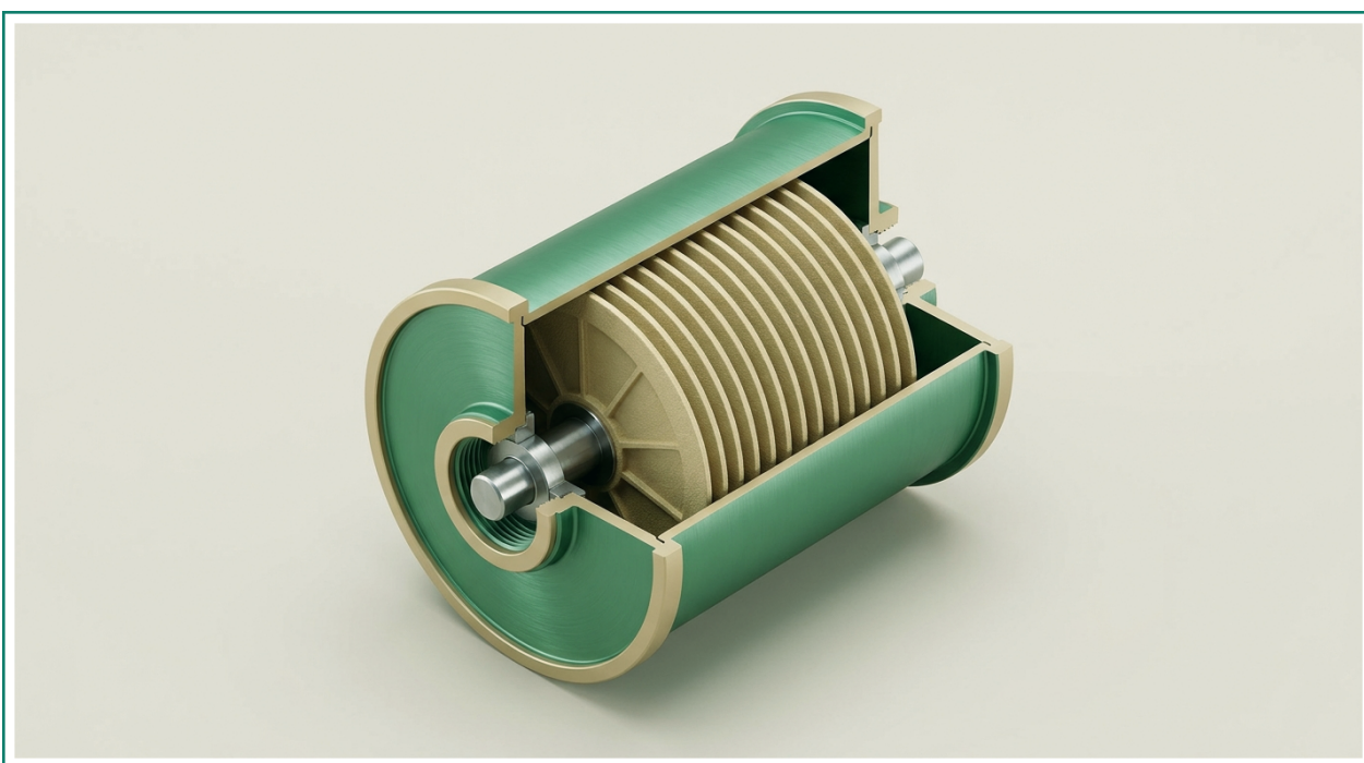
Батарея дисковых фильтров на общем коллекторе
