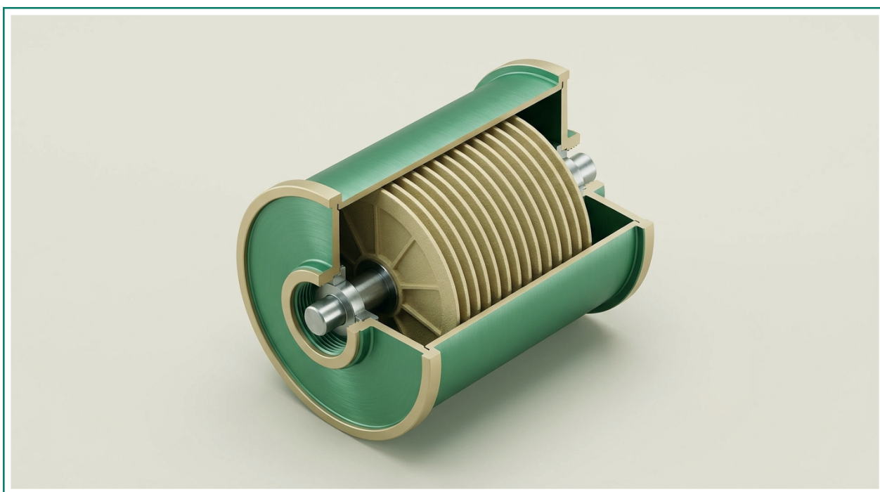
Стопка дисков дискового фильтра в разрезе
