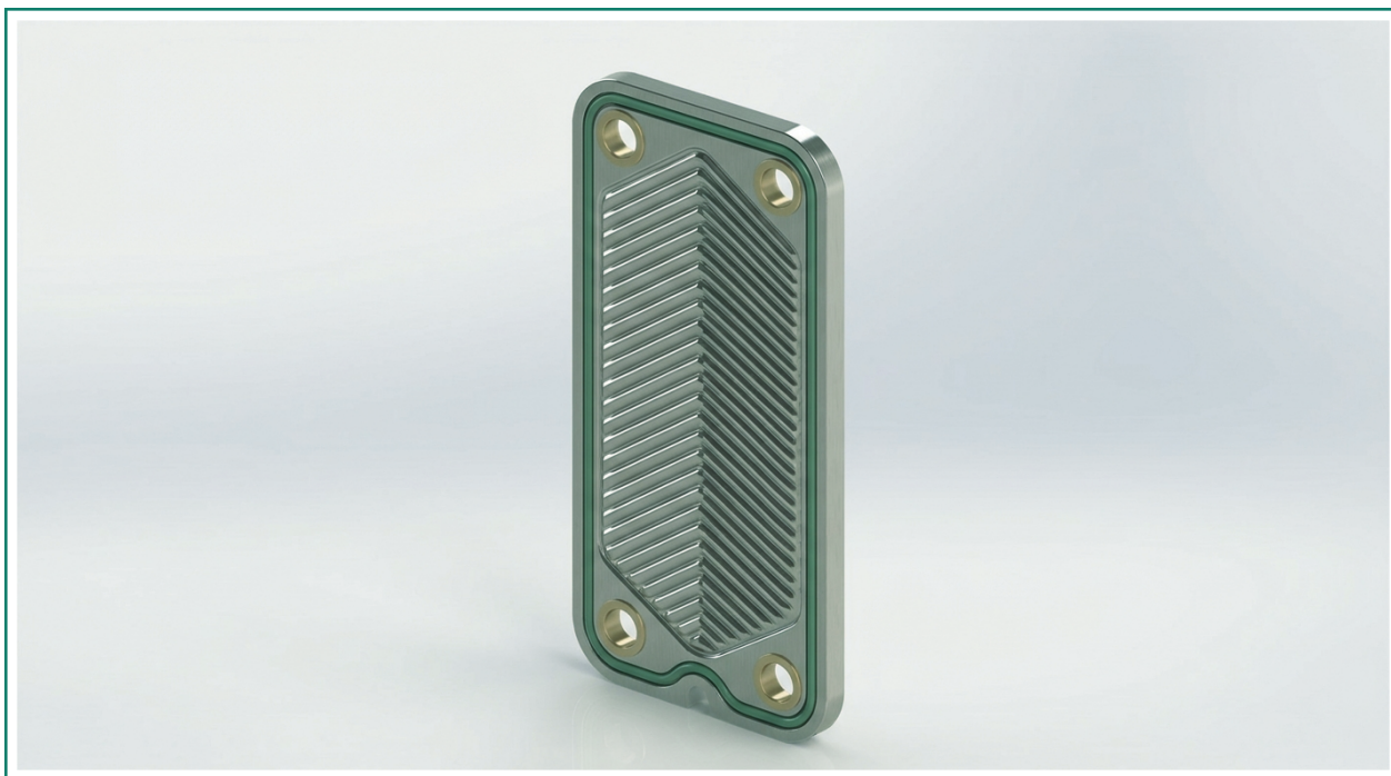
Пластина теплообменника: замеряют ширину, высоту и диаметр портов
