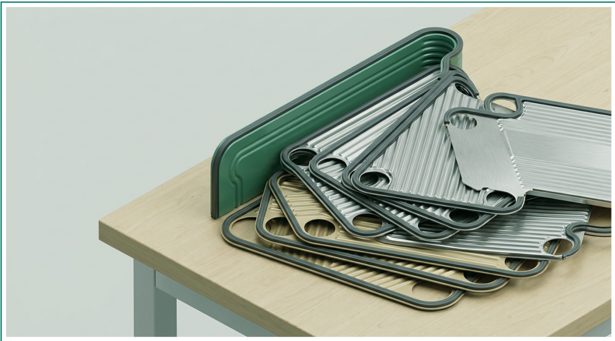
Комплект гофрированных пластин теплообменника Sondex
