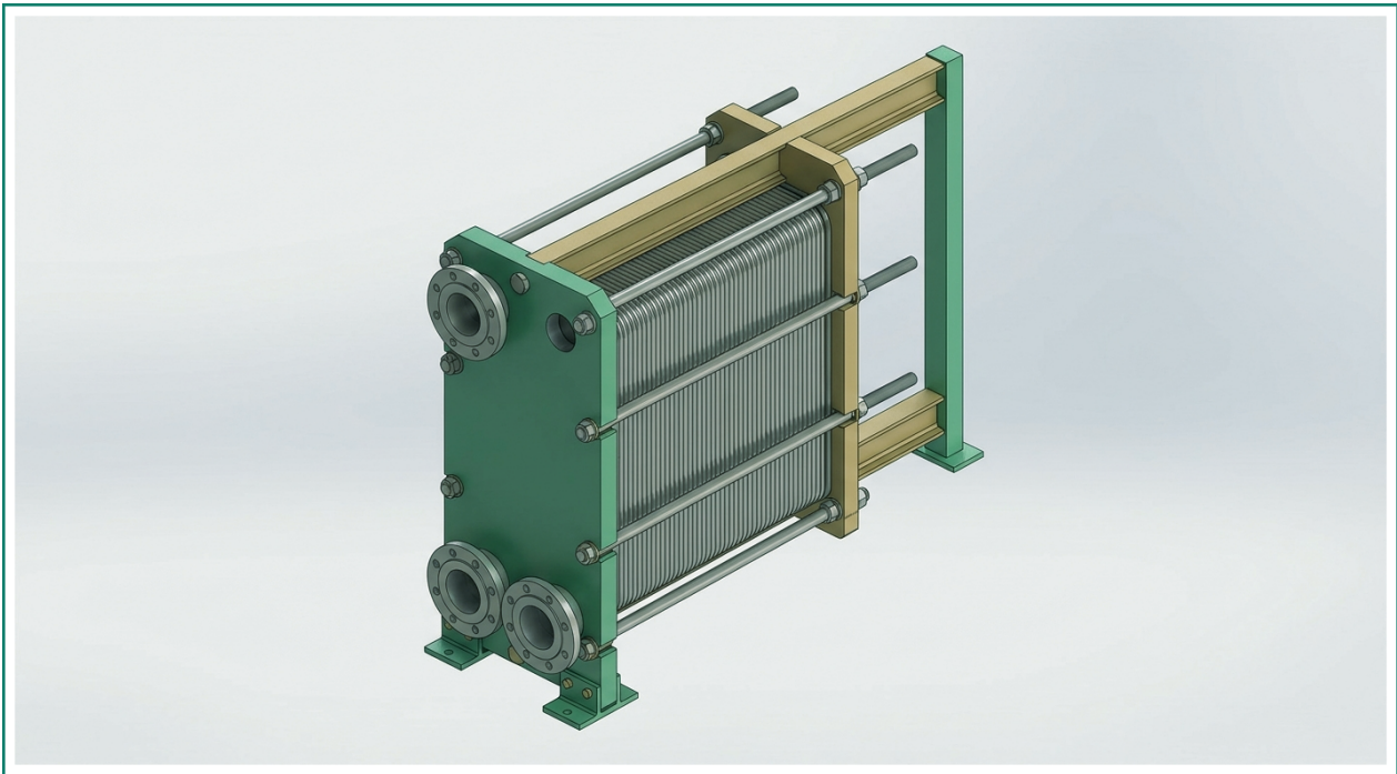
Разборный пластинчатый теплообменник линейки Funke GPL
