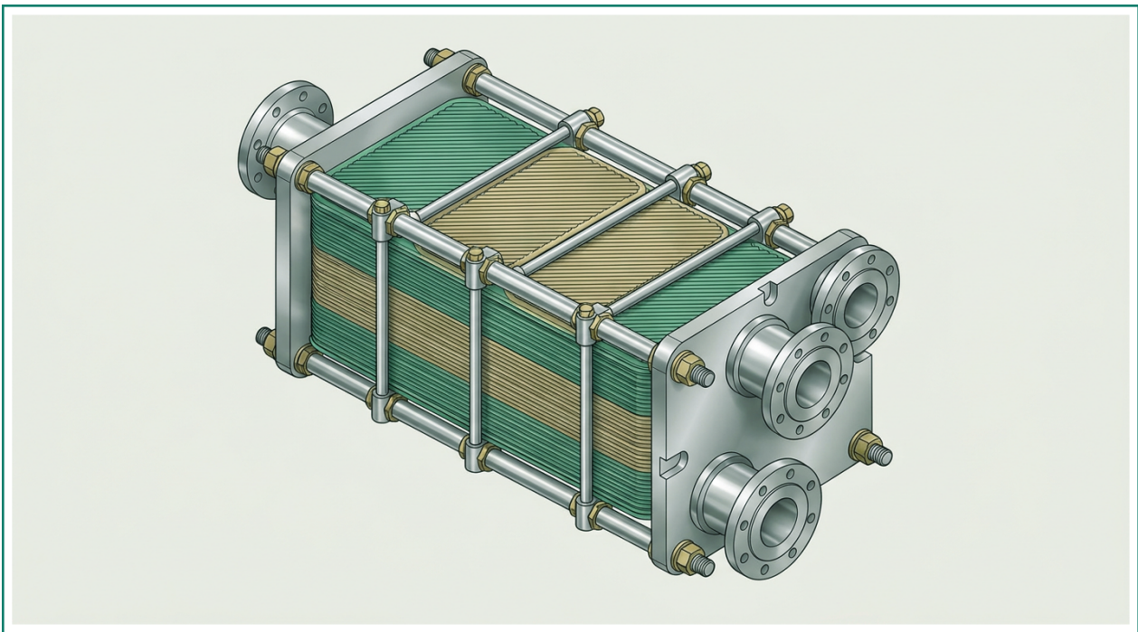
Полусварной теплообменник линейки Sondex SL
