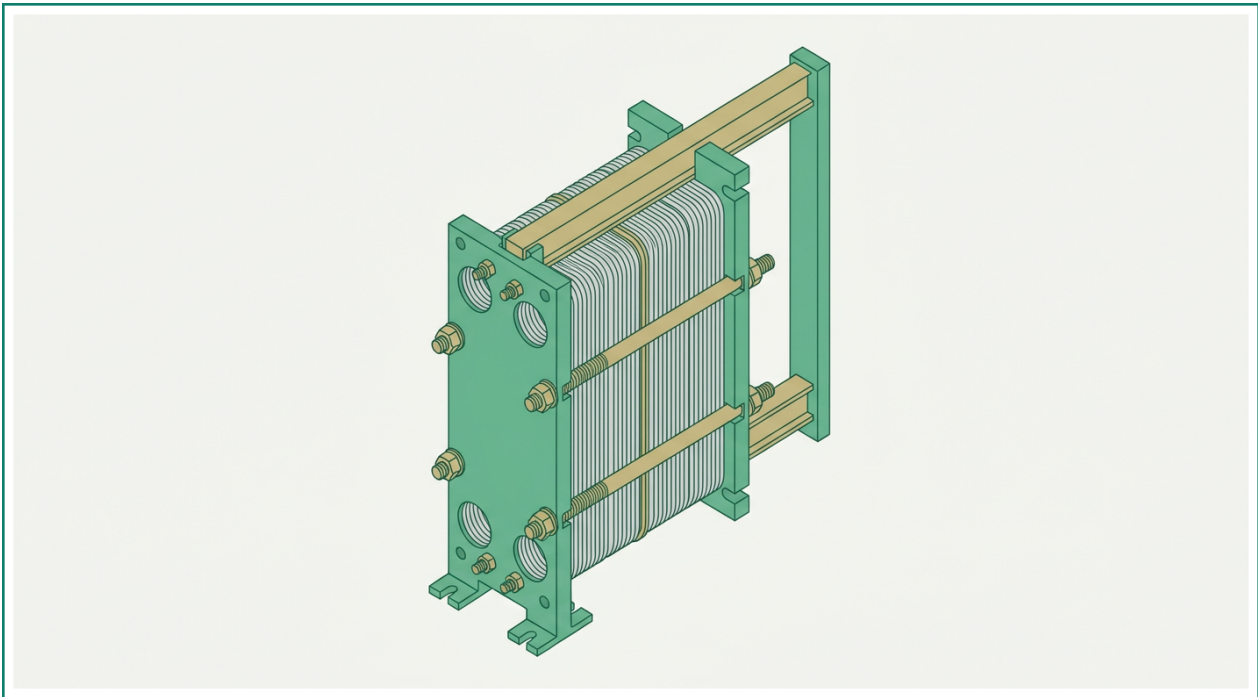
Разборный теплообменник линейки Kelvion GEA
