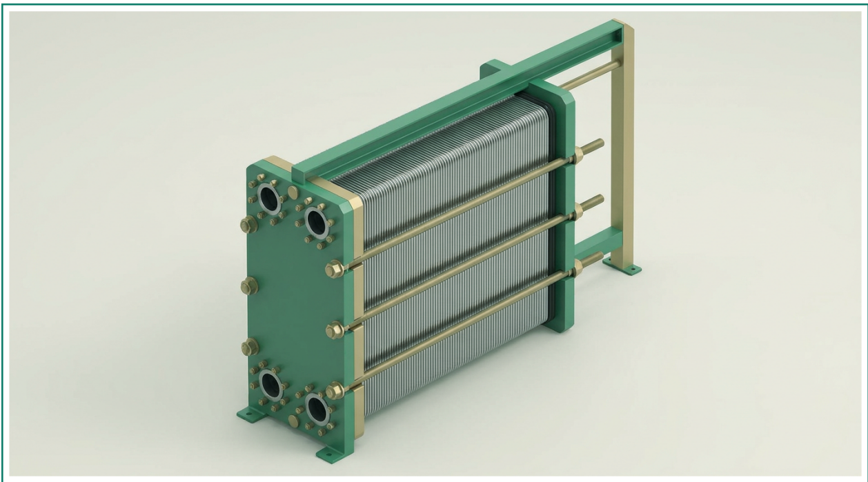
Разборный пластинчатый теплообменник линейки Ридан НН
